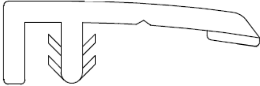
Die 1852 — 2-Part Start Edge Top
