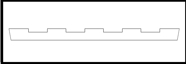
Die 1704 — PVC Stair Nosing
