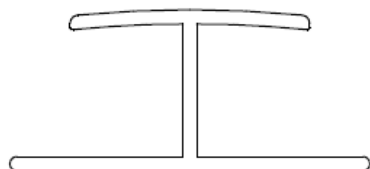
Die 1194 — 11mm—13mm 'H' Section
